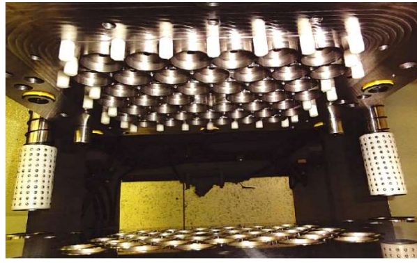
医療ゴム栓抜き金型
